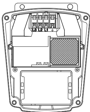
Fig. 4 Protection module
