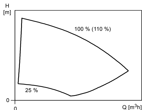
Fig. 18 Rango de trabajo de las bombas TPE Serie 2000
