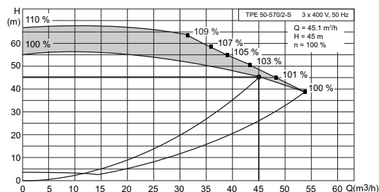
Fig. 19 Bombas TPE y TPED con curvas características ampliadas
